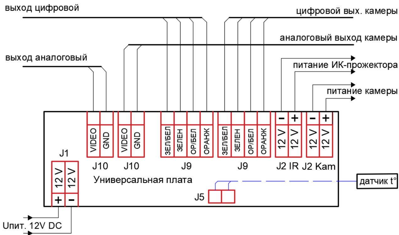
Рисунок 5б – Подключение исполнений 16
