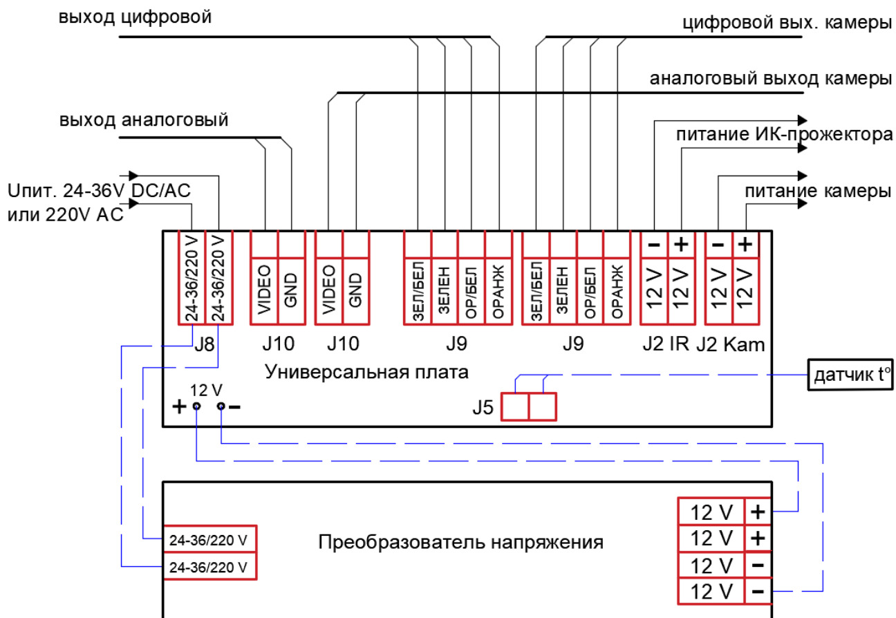
Рисунок 5а – Подключение исполнений 08; 09
