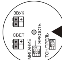
Рис.3 - Расположение клеммников и микропереключателей в коммутационном отсеке оповещателей «Плазма»Ех(м)-С3-40х20
