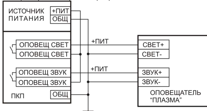
Рисунок 2 – Подключение оповещателя «Плазма»П-40х20 к релейным каналам оповещения приёмно-контрольного прибора.
