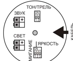
Рисунок 4 – Расположение клеммников и микропереключателей в коммутационном отсеке оповещателя «Плазма»П-С3-40х20
