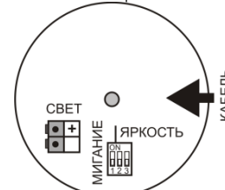
Рис.5 - Расположение клеммников и микропереключателей в коммутационном отсеке оповещателя «Плазма»П-С-40х20
