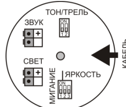
Рис.4 - Расположение клеммников и микропереключателей в коммутационном отсеке оповещателя «Плазма»П-С3-40х20
