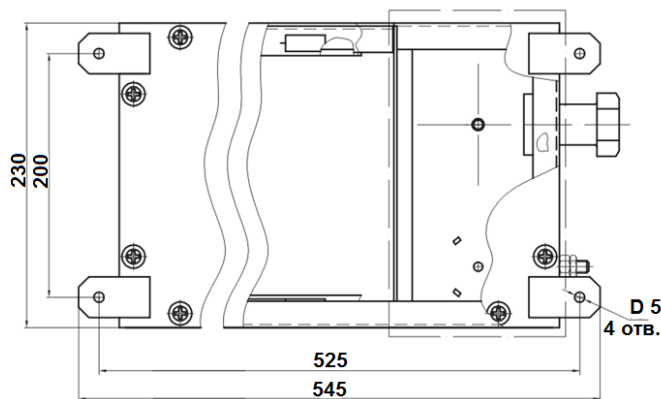
Рис3 - Габаритные и посадочные оповещателя «Плазма»П-40х20
