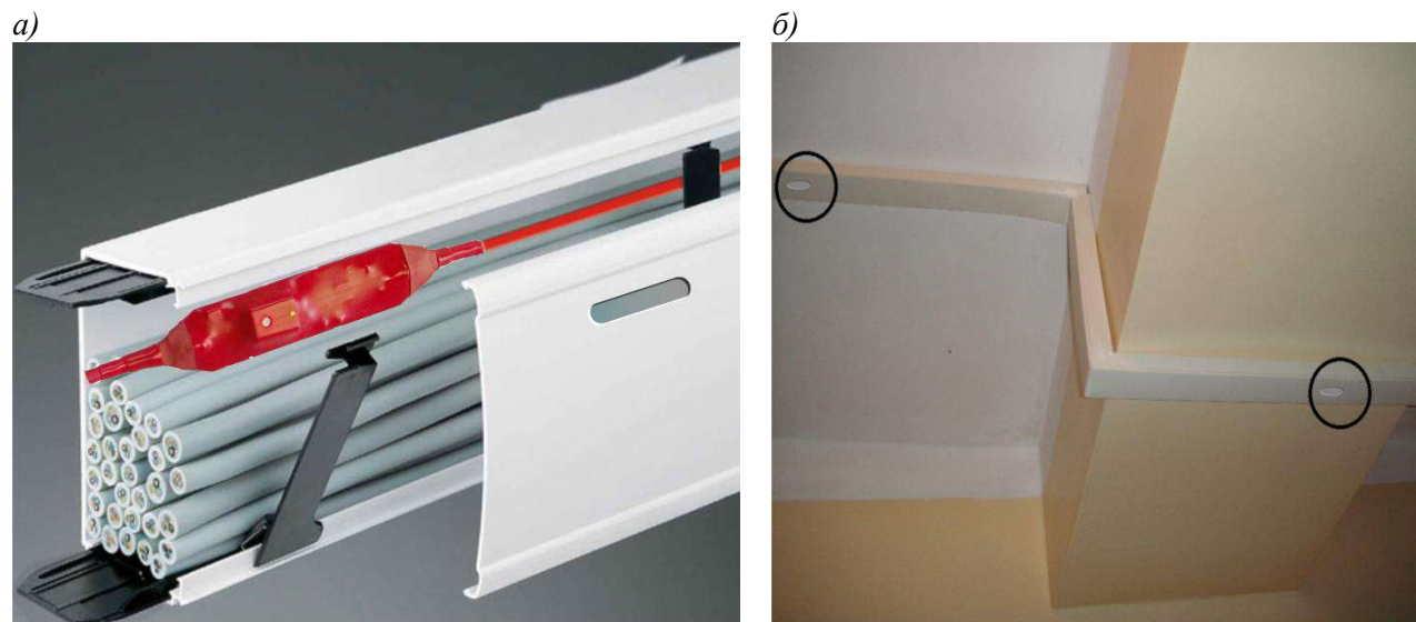
Рис.2.7. Внешний вид ЧЭ ProCab® , смонтированного в кабель-канале.
