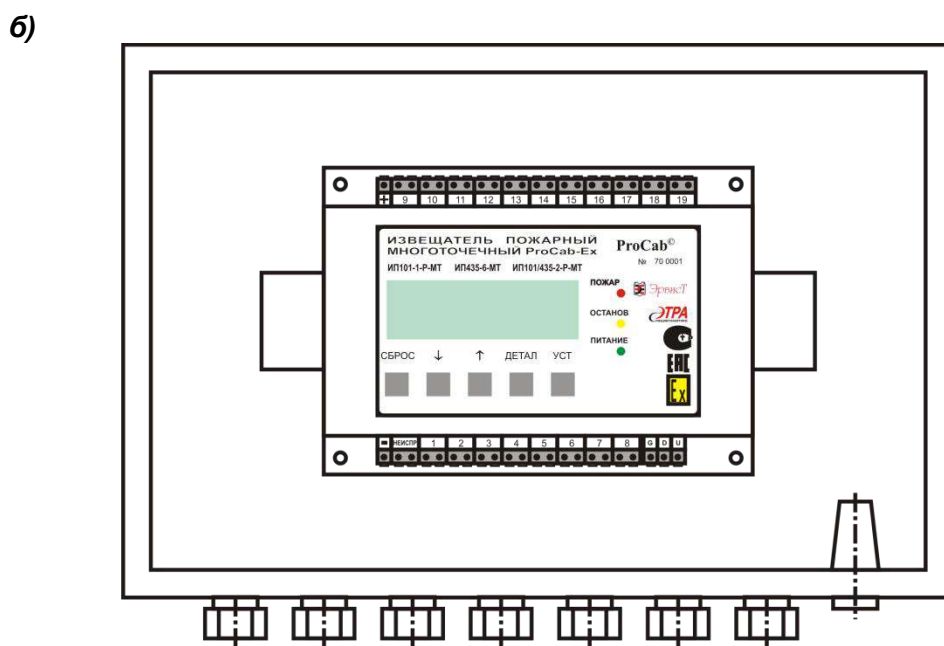
Рис.4.1. Внешний вид и габариты:
