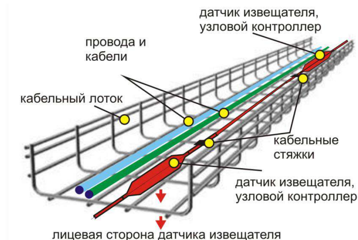
Рис.2.5. Прокладка ЧЭ ProCab® в решётчатых кабельных лотках.
