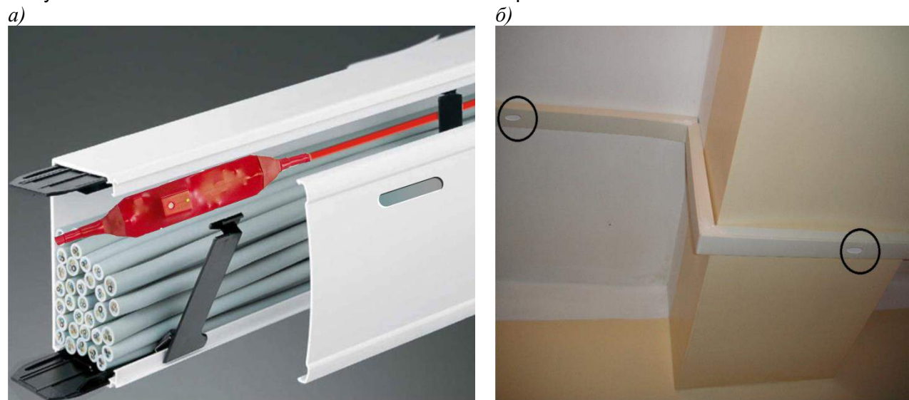
Рис.17. Внешний вид ЧЭ ProCab® , смонтированного в кабель-канале.
