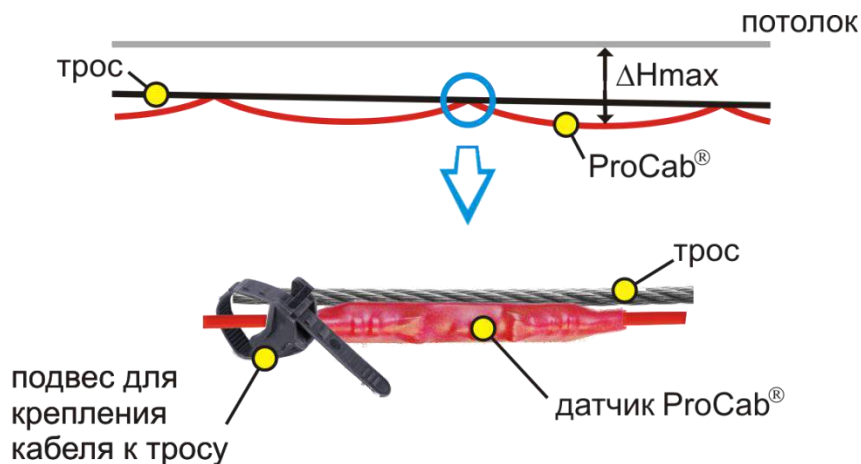
Рис.13. Монтаж ЧЭ ProCab® на тросу.
