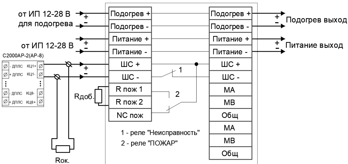
Рисунок 11 – Схема подключения к C2000-AP2 (AP-8) без использования режима «НЕИСПРАВНОСТЬ»
