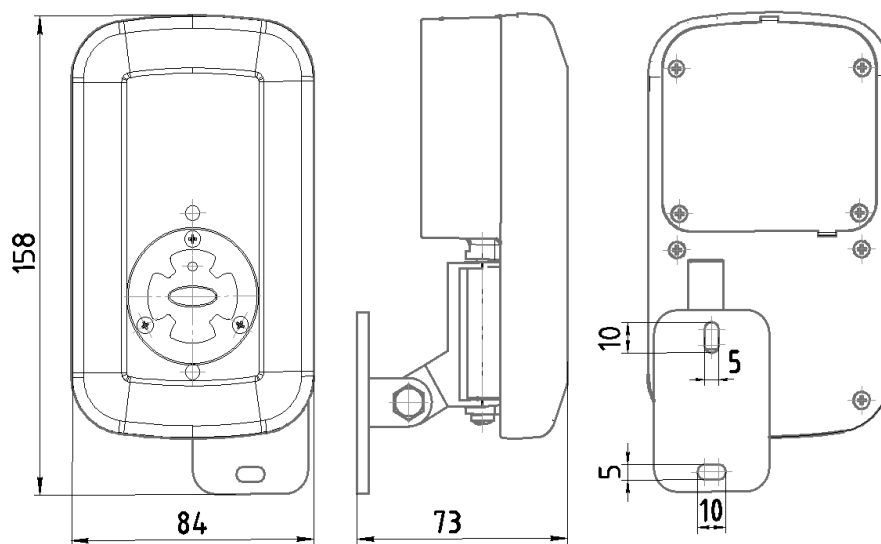
Рис. 1 – Сирин-Ехi-ИК+УФ-П-С, Сирин-Ехm-ИК+УФ-П-С
