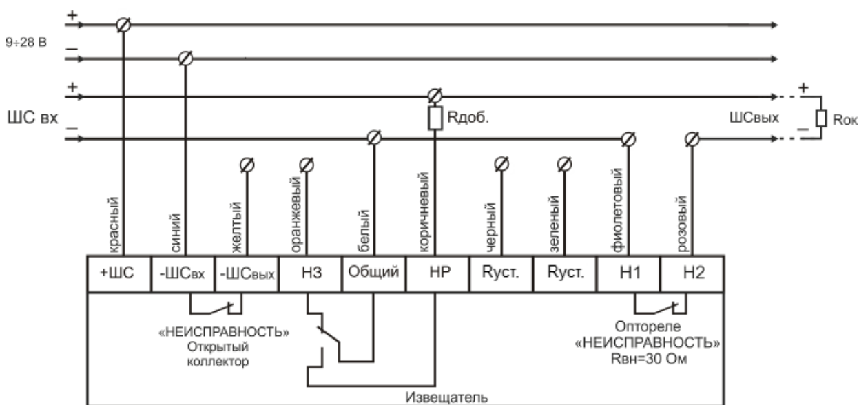
Рис. 6 – 4-х проводная схема подключения с использованием режима «НЕИСПРАВНОСТЬ»
