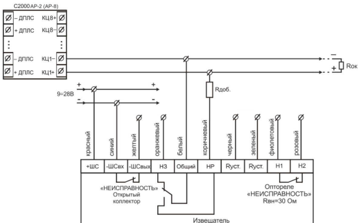
Рис. 9 – 4-х проводная схема подключения к С2000-АР2 (АР-8) без использования режима «НЕИСПРАВНОСТЬ»
