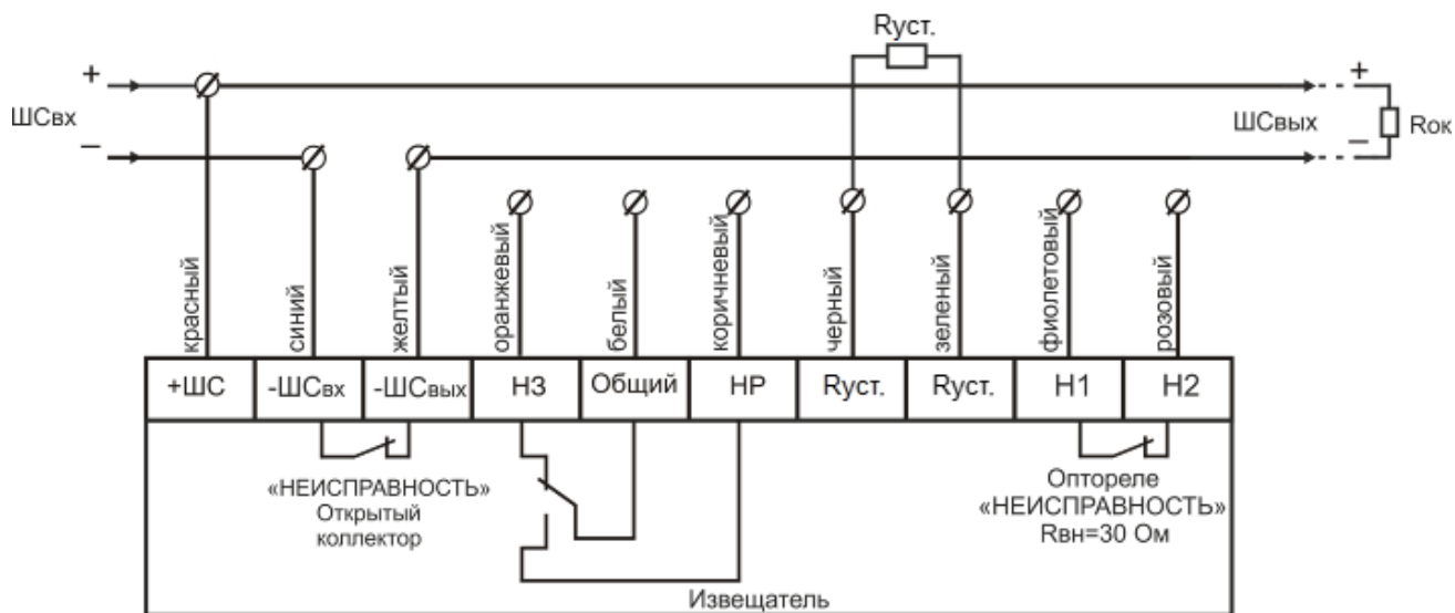
Рис. 4 – 2-х проводная схема подключения с использованием режима «НЕИСПРАВНОСТЬ»
