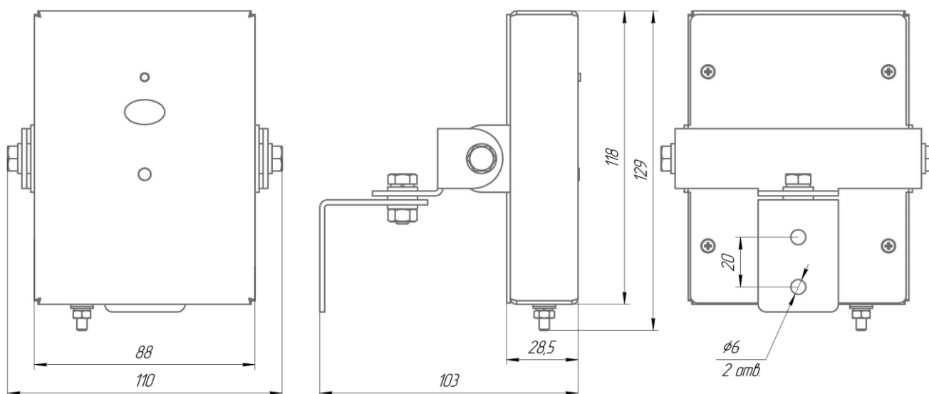
Рис. 2 – Сирин-Ехi-ИК+УФ-М-С, Сирин-Ехm-ИК+УФ-М-С, Сирин-Ехi-ИК+УФ-Н-С, Сирин-Ехm-ИК+УФ-Н-С
