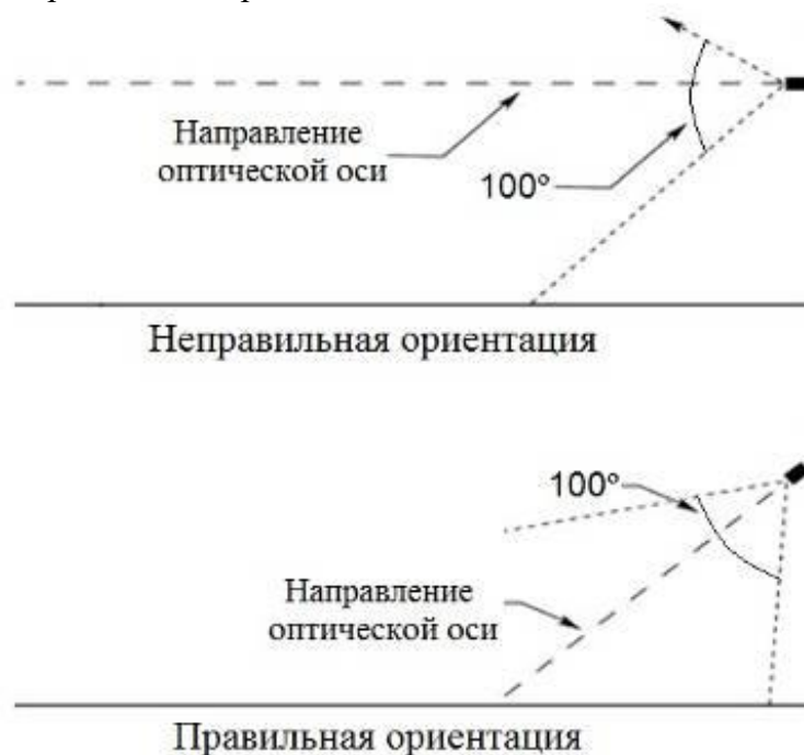
Рис. 3 – Установка извещателя по отношению к горизонту
