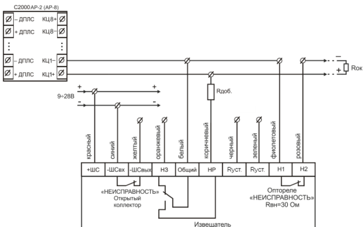
Рис. 8 – 4-х проводная схема подключения к S2000-AP2 (AP-8) с использованием режима «НЕИСПРАВНОСТЬ»
