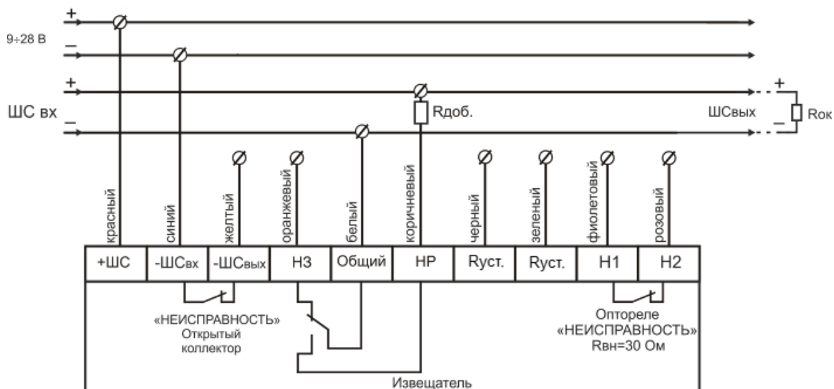
Рис. 7 – 4-х проводная схема подключения без использования режима «НЕИСПРАВНОСТЬ»
