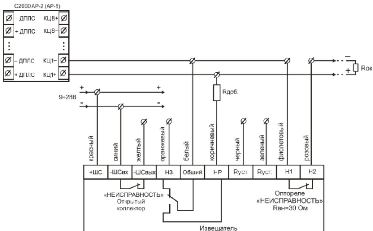
Рис. 8 – 4-х проводная схема подключения к С2000-АР2 (АР-8) с использованием режима «НЕИСПРАВНОСТЬ»
