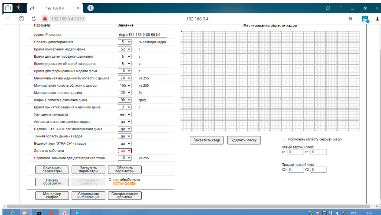
Рисунок 13 – Установка параметров ИПВ в web-интерфейсе.
