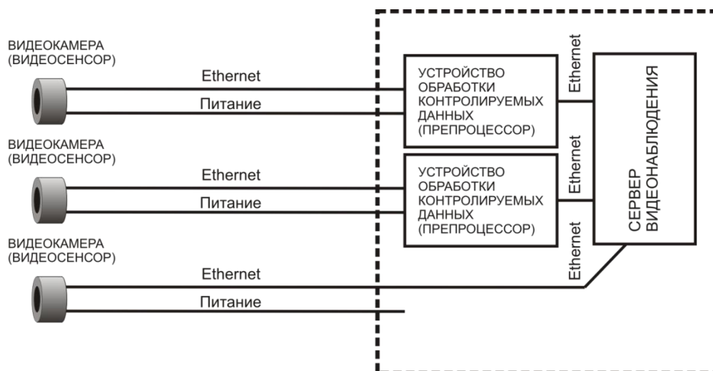
Рисунок 43 – Подключение нескольких ИПВ к серверу видеонаблюдения
