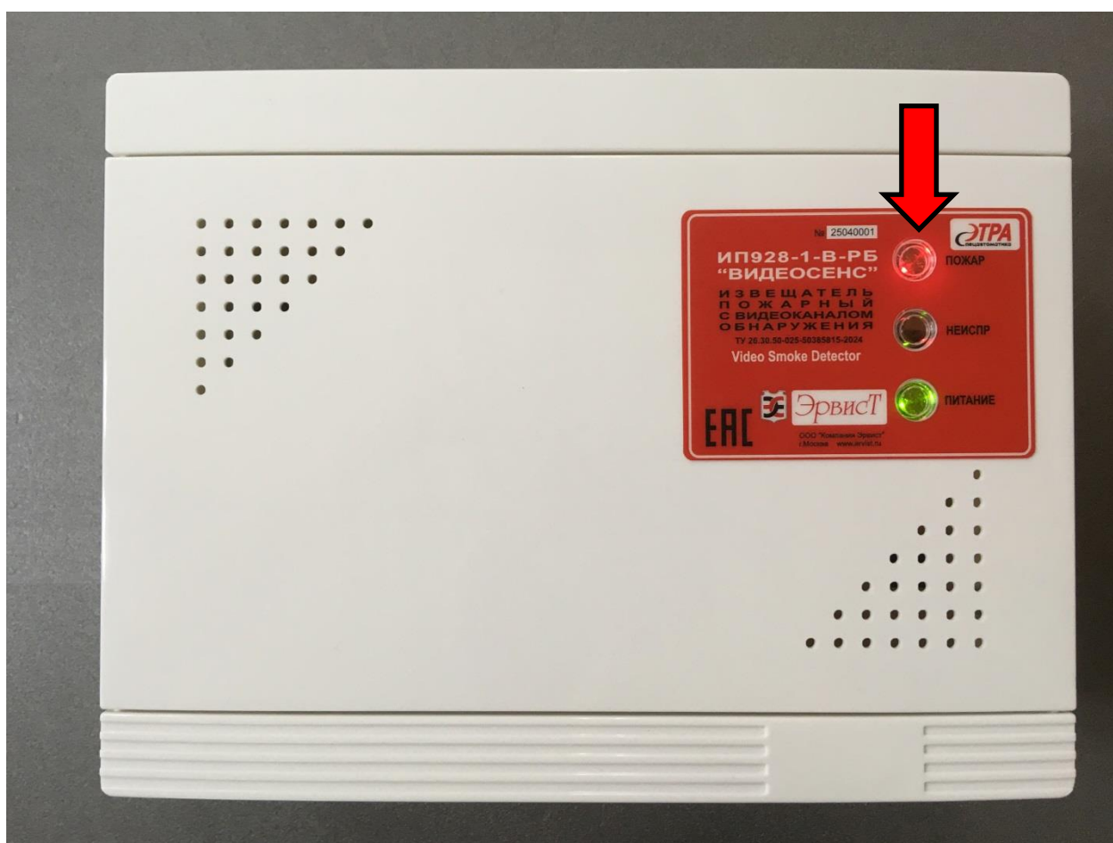
Рисунок 19 – Индикация УКОД при обнаружении пожара.
