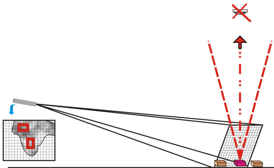
Рисунок 11 – Направление видеосенсора для определения пожара непосредственно на открытой площадке.
