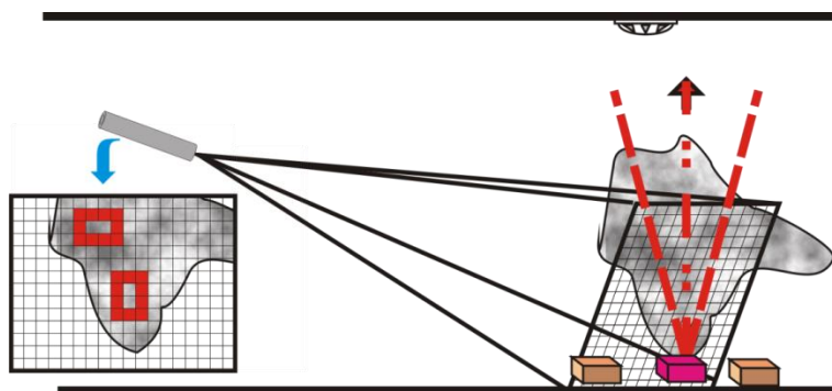
Рисунок 10 – Направление видеосенсора для определения пожара непосредственно на полу помещения с высокими потолками.
