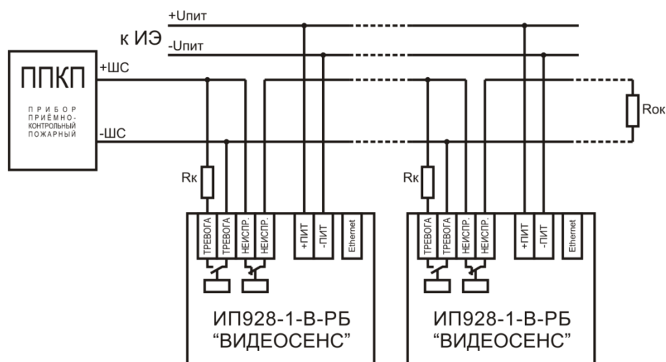
Рисунок 12 – Подключение ИПВ «Видеосенс» в шлейф ППКП.
