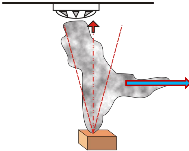
Рисунок 2 – Для срабатывания извещателей конвективного типа необходим контакт между чувствительной системой извещателя и продуктами горения.
