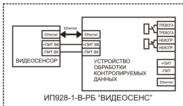
Рисунок 6 – Структура ИПВ и подключения к нему.
