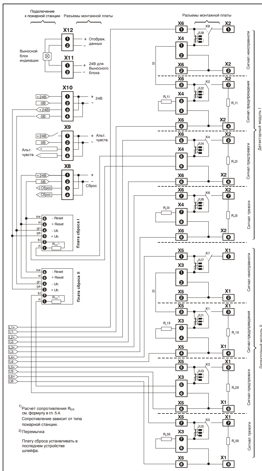
Рис. 5.12: Пример подключения TITANUS TOP · SENS® к ПКП с платой сброса
