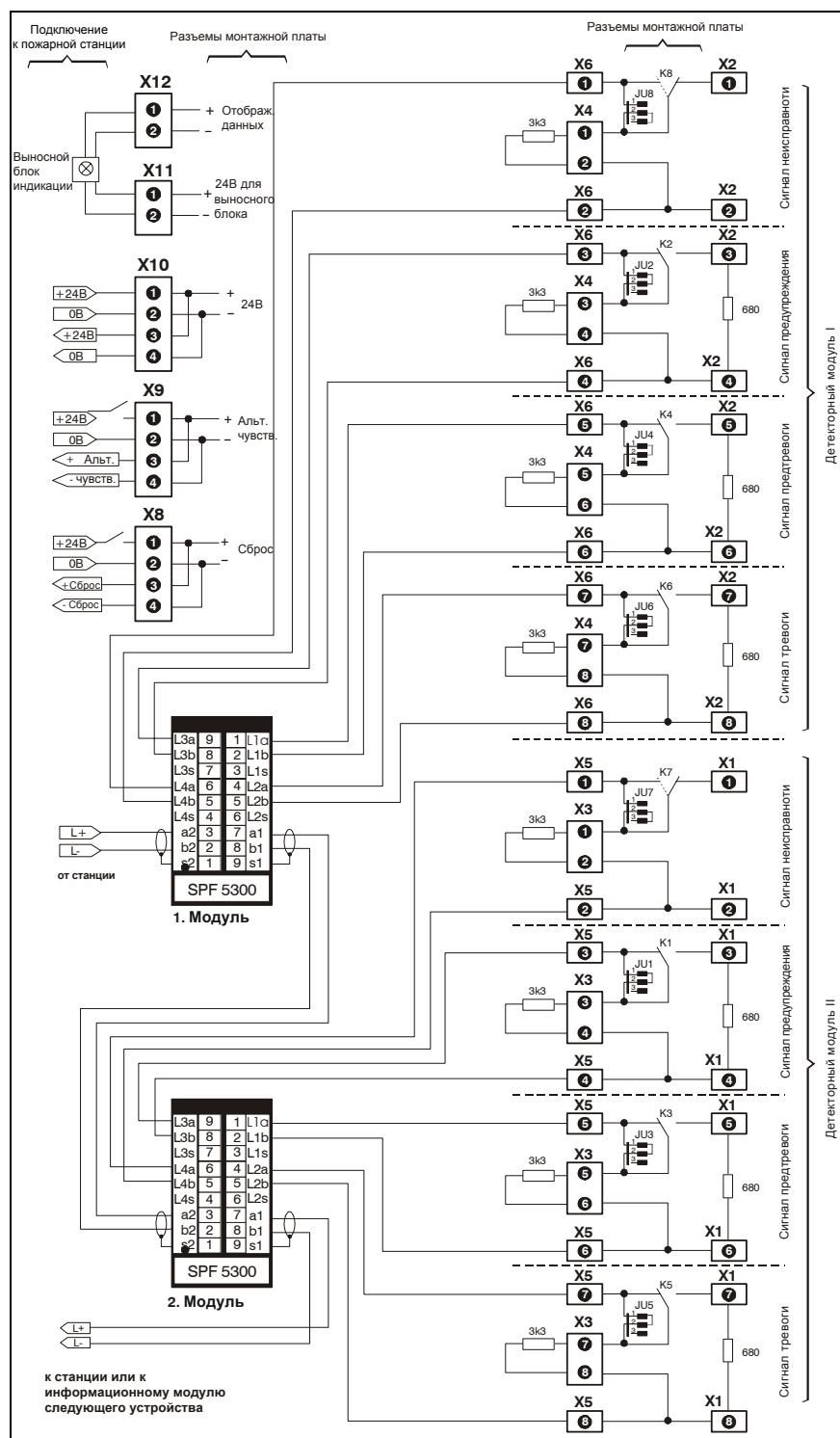
Рис. 5.19: Подключение информационного модуля SPF 5300 и TITANUS TOP · SENS®
