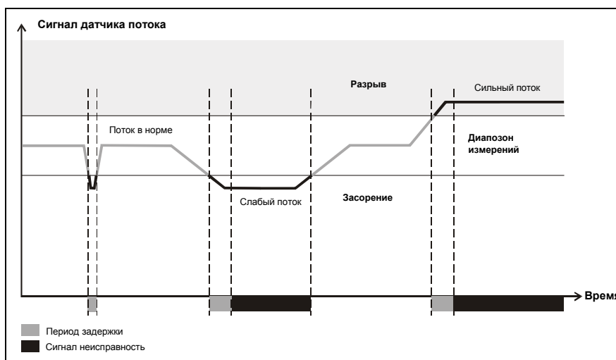
Рис. 2.2: График сигнала при формировании неисправности датчика потока
